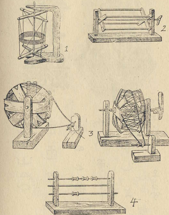
Resim: 103. Nohurlu Türkmenlerinde çıkık ve ip bükme aletleri.
