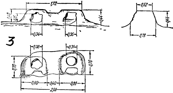
Resim: 27 1). Doğü Türkistan'da fûrk tandır. 2). Kara-Kalpak Türklerinin eski ocak ve tandırları.
