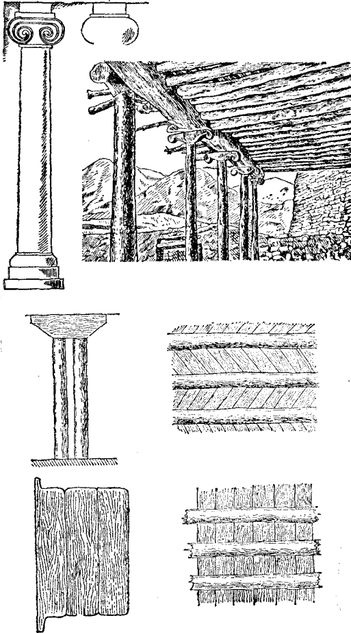
Resim: 52. Nohurlu Türkmenlerinde ayvan yapısı ve ağaç çatmaları.
