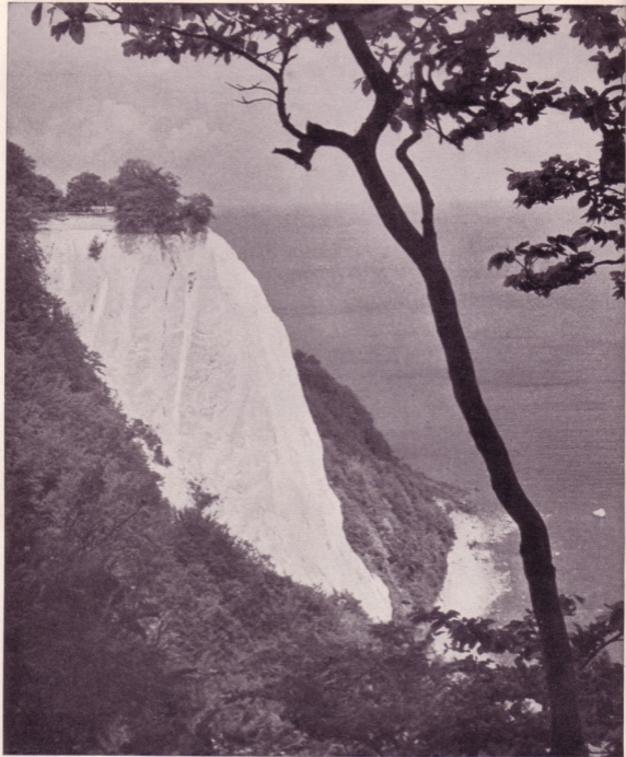
KREIDEFELSEN VON STUBBENKAMMER / INSEL RÜGEN
