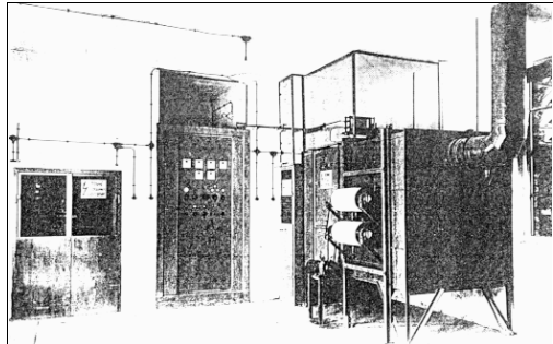
Photos der stationären Kurzwellenentlausungsanlage im BW 160 des KL Auschwitz 1944
