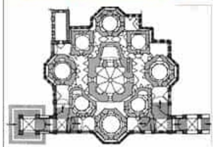
Покровский собор (план собора)
