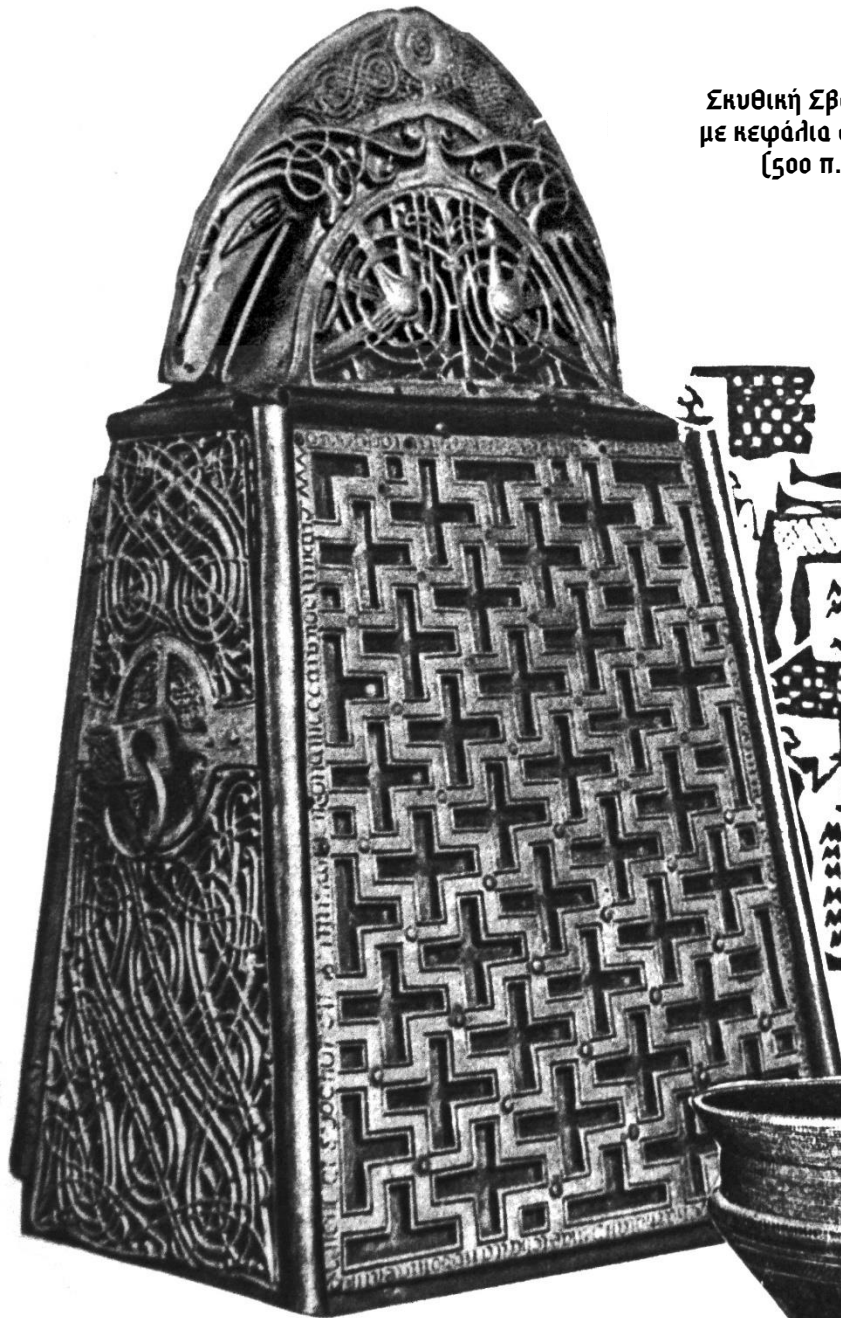
Το εθνικό κειμήλιο της Ιρλανδίας: η λάρνακα του Αγίου Πατρίκιου (σταυρός, Σβάστικα και το Δέντρο της Ζωής άνωθέν τους)
