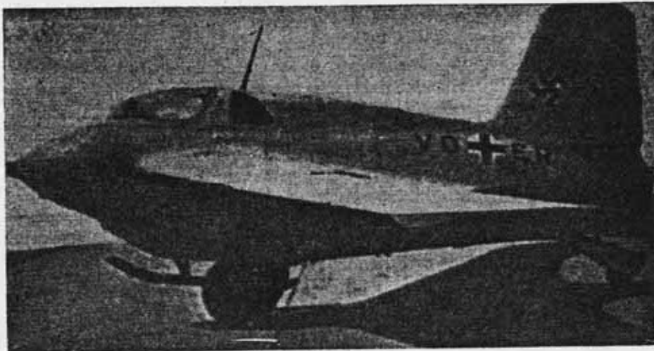
Me-163; ascendía 13.000 metros en tres minutos. Dirigido por un piloto radioeléctrico accionado desde tierra. Iba a entrar en acción a mediados de 1945. Demasiado tarde. . .
