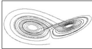
Proyección de un Atractor de Lorenz tridimensional
