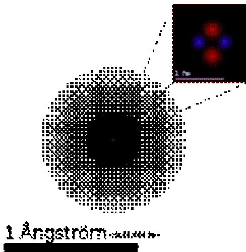
Fotografía de un átomo de helio.
