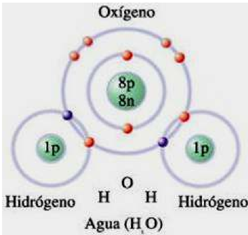
Composición molecular del agua.
