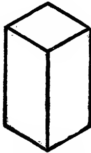
FIG. 12.—DOUBLE CUBE.
