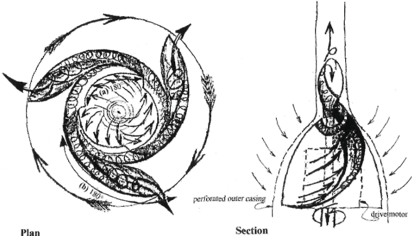
Fig. 12: 3-blade Bioturbine
