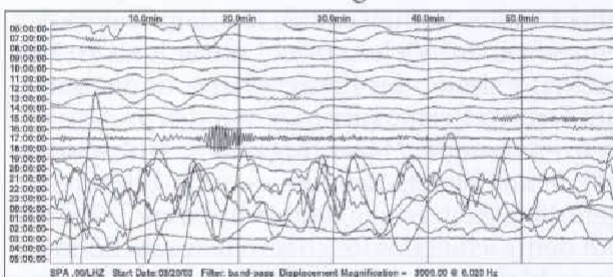
Angebliches Seismogramm einer amerikanischen Atombombenzündung am 20. März 2003 in Neu-Schwabenland
