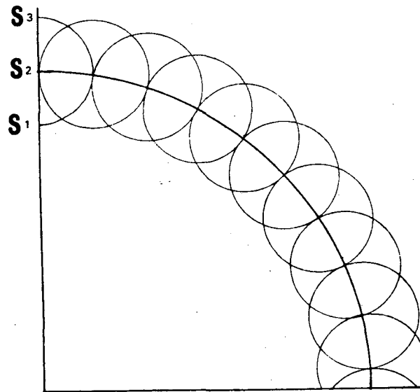
PROPAGACION DE UNA ONDA SEGUN EL PRINCIPIO DE HUYGENS.
